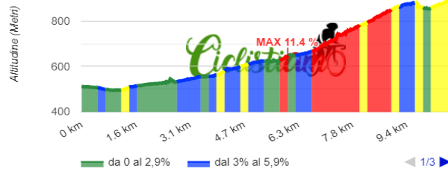
altimetria tratto VILLANOVA M. - FRABOSA SOPRANA KM. 10,7
